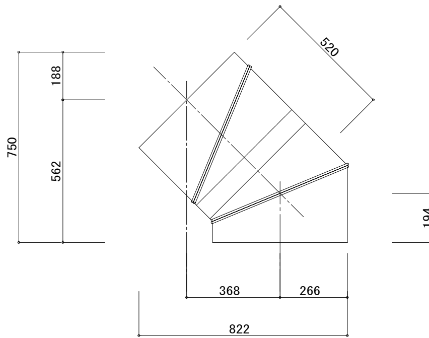
45° アンゲル SCALE 1:15
