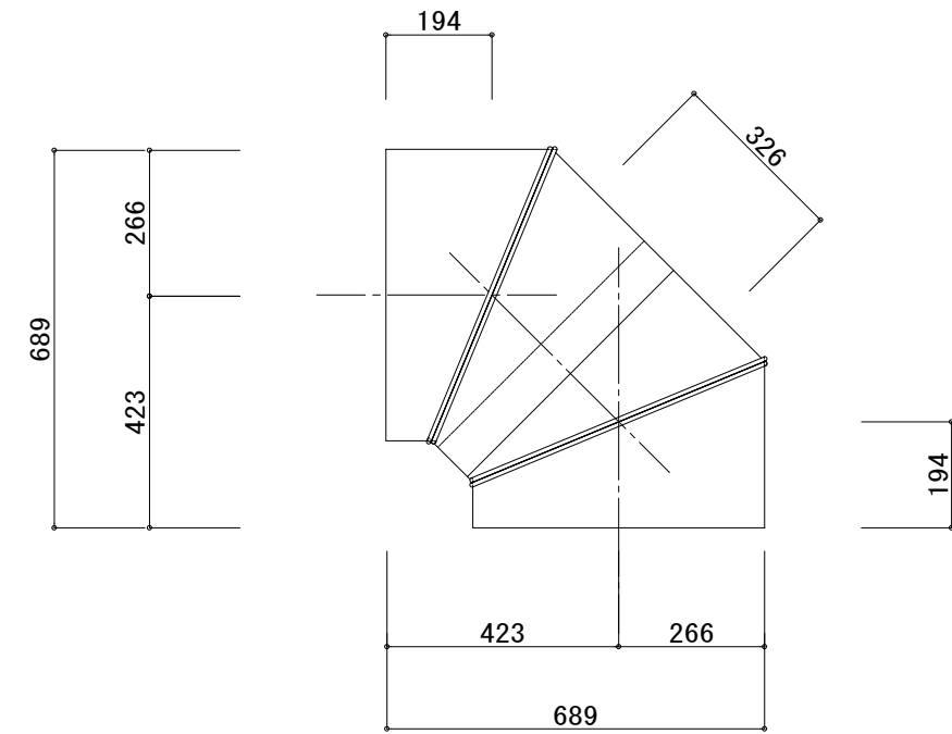
90° アンゲル SCALE 1:15
