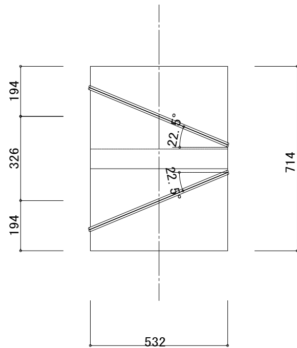
ストレート SCALE 1:15
