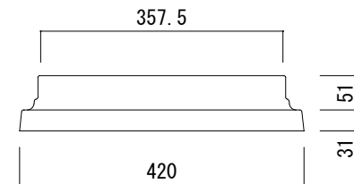
アジャストリング
