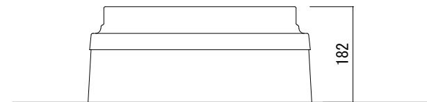
アジャストリング取付後ルーフベース高さ
