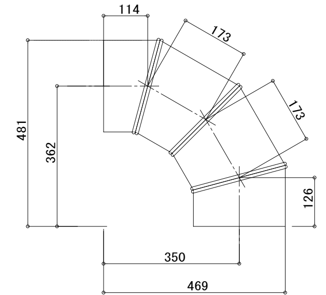
90° アングル SCALE 1:10
